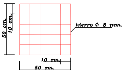
DETALLE - C PARRILLA p/Base De Pilar (Item 2)
