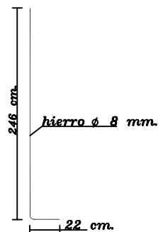
DETALLE - B (Item 2)
