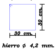
DETALLE - A Del Estribo: (Item 1)
