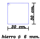
DETALLE - A Del Estribo: (Item 1)
